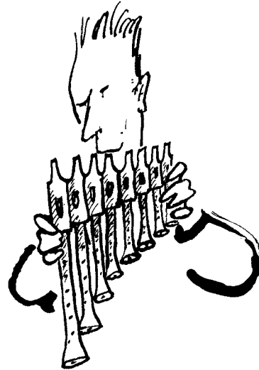
Panflöte (Hilbert)
